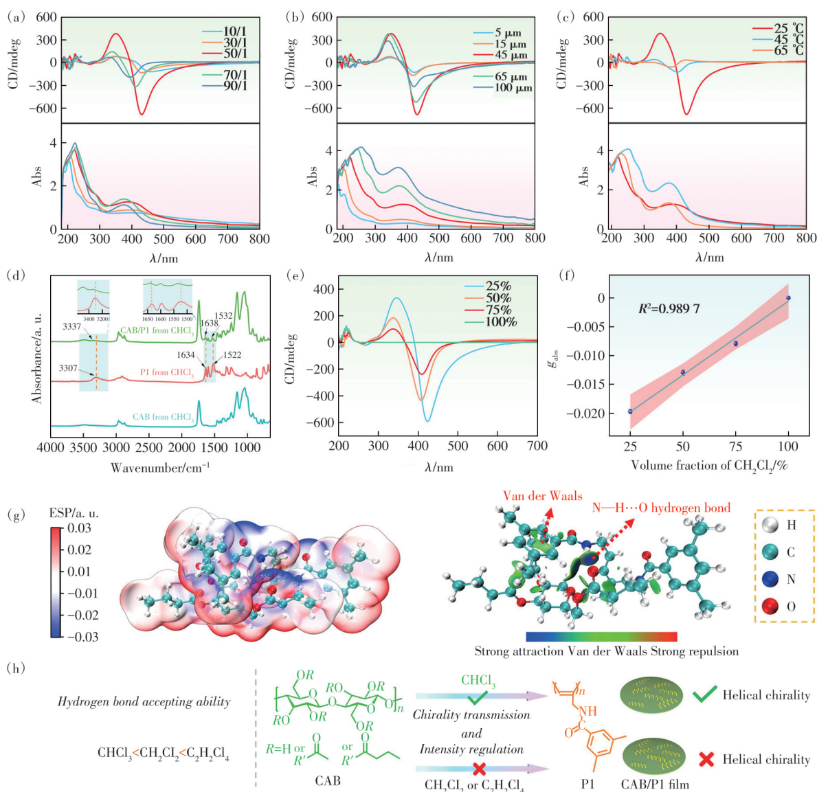
图4 (a)~(c)不同CAB/P1质量比、不同厚度、不同成膜温度下CAB/P1薄膜的圆二色性(CD)与紫外-可见(UV/Vis)光谱; (d)来自CHCl 3 的CAB薄膜、P1粉末及CAB/P1薄膜的傅里叶变换红外(FT-IR)光谱; (e)不同CHCl 3 /CH 2 Cl 2 混合物中CH 2 Cl 2 体积分数下获得的CAB/P1薄膜CD光谱; (f)CAB/P1薄膜 g_{abs} 值与CHCl 3 /CH 2 Cl 2 混合物中CH 2 Cl 2 体积分数的关系; (g)CAB/P1复合物的ESP分布图及CAB与P1间分子间相互作用的IGMH分析; (h)溶剂依赖性手性传递示意图 [60]
