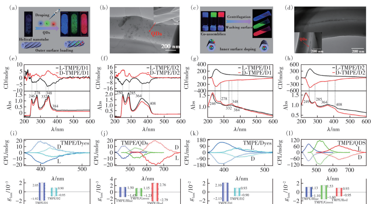
图 6 (a)手性螺旋纳米管外表面负载非手性量子点过程示意图;(b)透射电子显微镜观察到量子点负载于纳米管外表面;(c)手性螺旋纳米管内表面掺杂非手性量子点过程示意图;(d)透射电子显微镜观察到量子点掺杂于纳米管内表面;(e)、(f)、(i)手性螺旋纳米管外表面诱导的染料 D1 与 D2 的 CD 光谱及 CPL 光谱;(j)手性螺旋纳米管外表面诱导三种不同颜色染料的 CPL 光谱;(g)、(h)、(k)手性螺旋纳米管内表面诱导的染料 D1 和 D2 的 CD 光谱及 CPL 光谱;(l)手性螺旋纳米管内表面诱导三种不同颜色染料的 CPL 光谱 [66]
