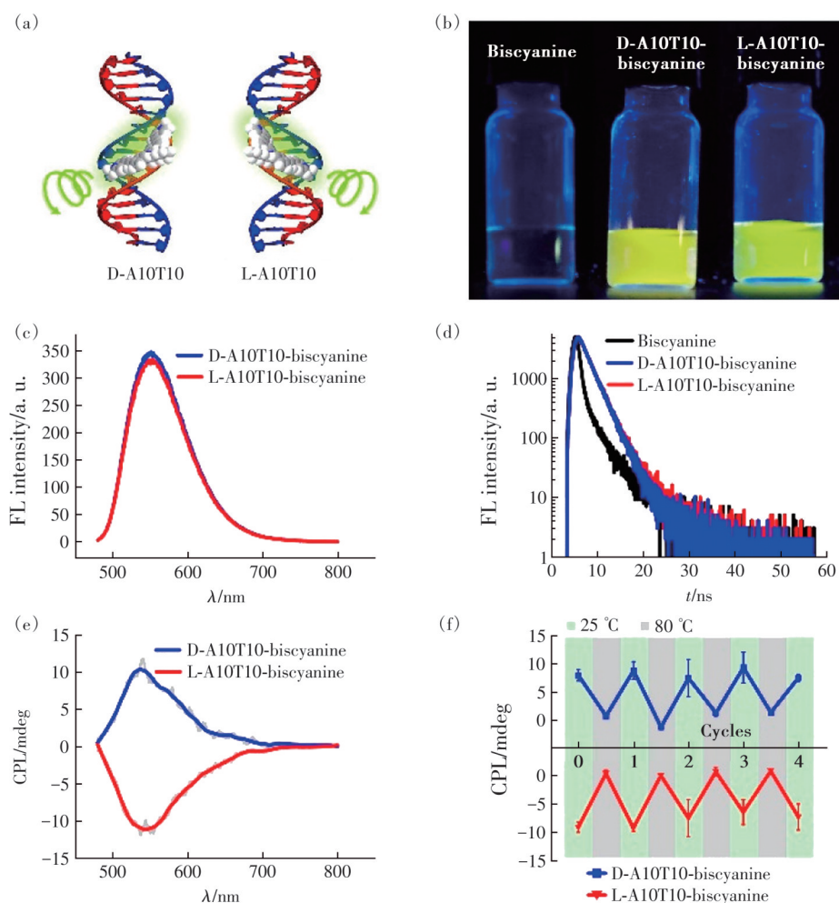
图3 (a)DNA双链-双氰胺复合材料示意图;(b)紫外照射下DNA双链-双氰胺复合材料的图像;(c)D-与L-DNA双链与双氰胺分子协同组装后的对映异构体的荧光光谱;(d)D-与L-DNA双链与双氰胺分子协同组装后的对映异构体的荧光衰减曲线;(e)D-与L-DNA双链-双氰胺对映异构体的镜像CPL光谱;(f)循环热处理后对映异构体的圆偏振光谱 [59]
