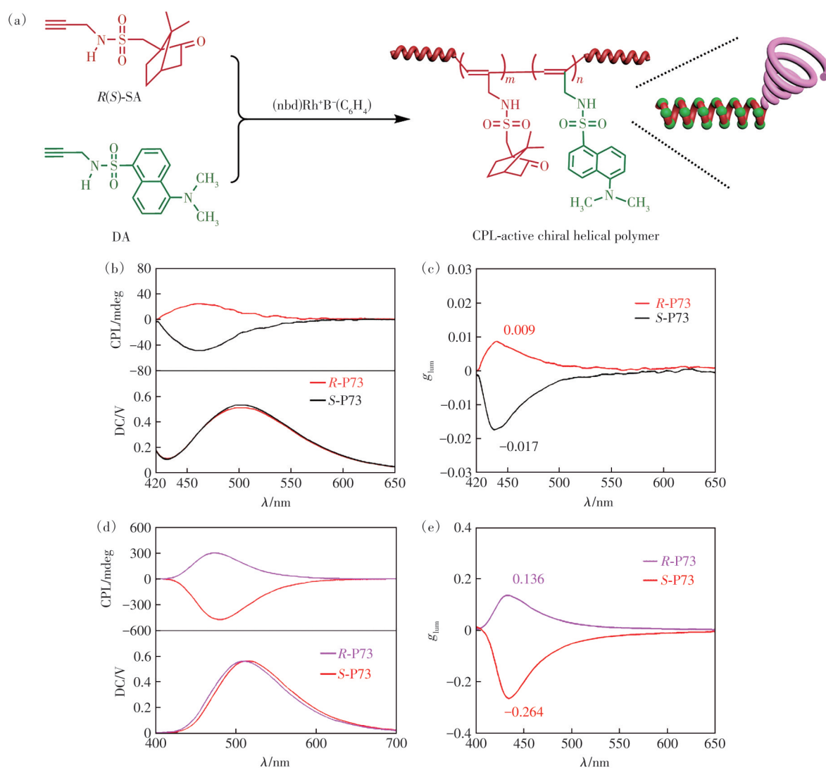
图2 (a)制备具有CPL性能的荧光手性螺旋单取代聚乙炔;(b)、(d) R -P73和 S -P73在CHCl 3 溶液中经369 nm激发产生的CPL光谱;(c)、(e) R -P73和 S -P73经369 nm激发时CPL不对称因子 g_{lum} 随波长的变化曲线。在(b)和(d)中, [R-P73]=[S-P73]=1 mmol/L;在(c)和(e)中, [R-P73]=[S-P73]=10 mmol/L [47]
