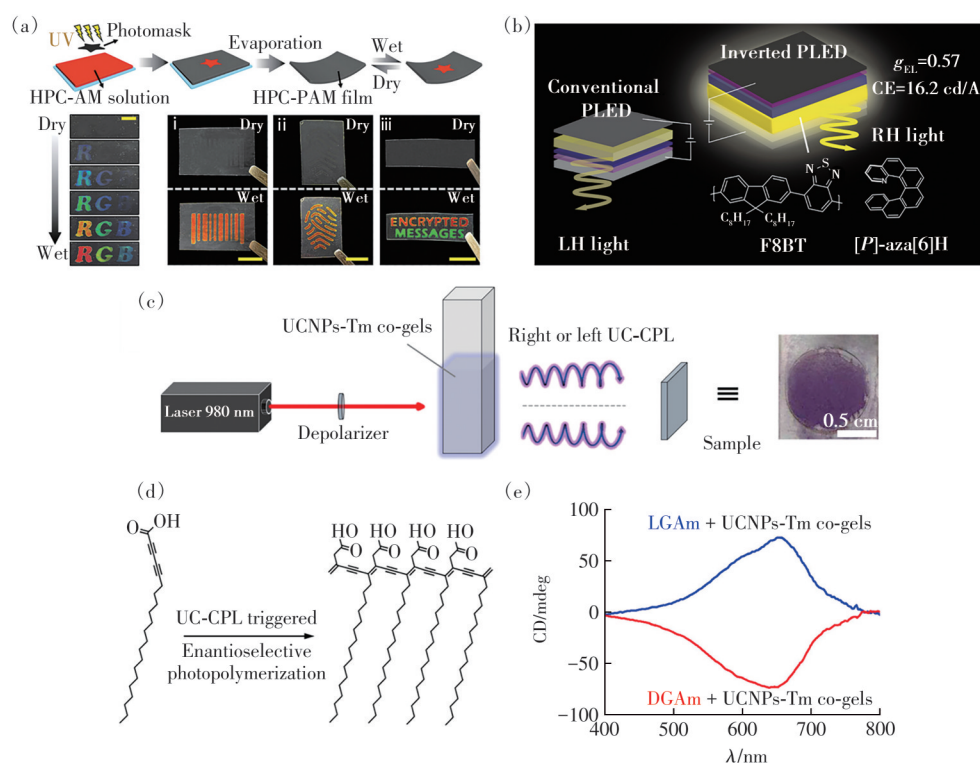
图 7 (a)制备带有隐藏图案的 HPC-PAM 薄膜,以及多色图案从干燥状态到湿润状态逐步显现隐藏信息过程 [73] ; (b)器件具有高 g_{EL} 与高电流效率用于 CP-OLEDs [79] ; (c)HA 对映选择性光聚合装置示意图; (d)HA 聚合示意图; (e)经 UCNPs-Tm 掺杂手性脂质凝胶产生的 CPL 照射后 PDA 薄膜的圆二色性光谱 [82]
